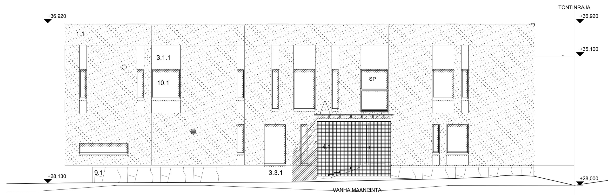
JULKISIVU ITÄÄN
